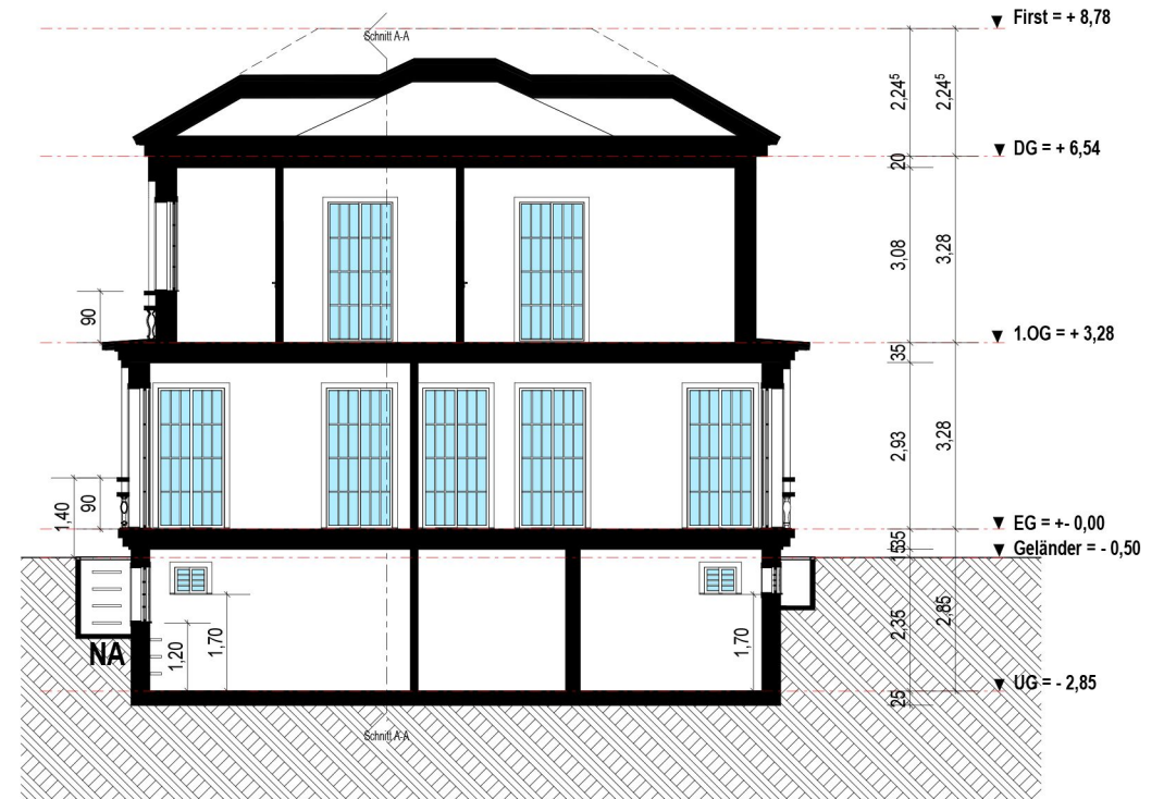
LÄNGSSCHNITT
