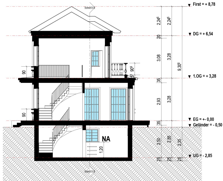
QUERSCHNITT
